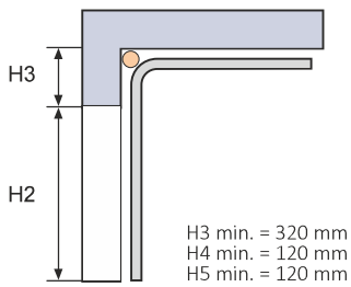
RÉDUIT IND-RL
