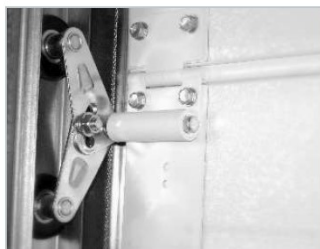
Système roulettes duplex
