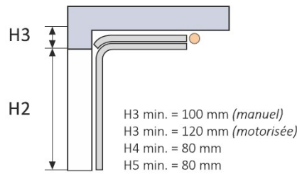
RÉDUIT RES100
