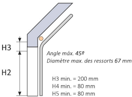
INCLINÉ RES200i
